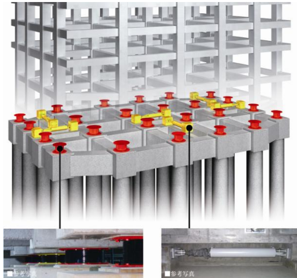
＜積層ゴム＞
